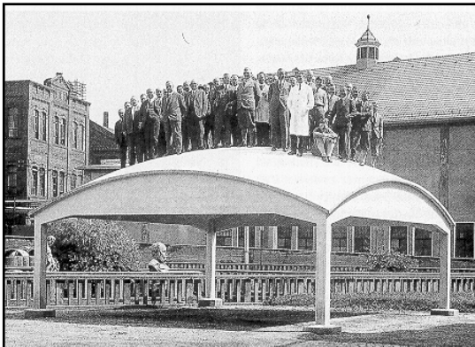
Toiture expérimentale, Jena, 1932, ing. F. Dischinger, \ell = 7 \times 7 \text{ m}
