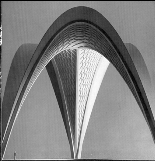
Projet de cathédrale à New Norcia, Australie Arch. P.L. Nervi, A. Nervi, F. Vacchini, C. Vannoni
