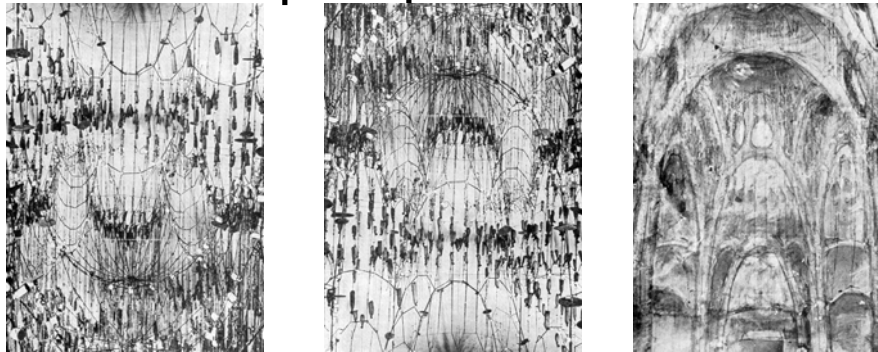
Maquette funiculaire et esquisse de la structure de la chapelle Güell à Barcelone, 1898-1915, arch. A. Gaudí
