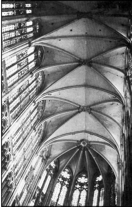
Cathédrale de Beauvais, 1337
