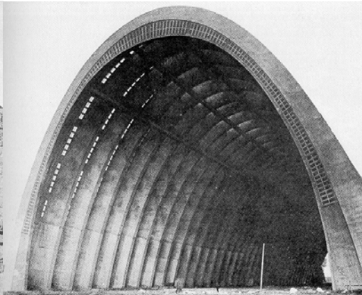
Hangar pour dirigeables, Orly, 1923, ing. E. Freyssinet
