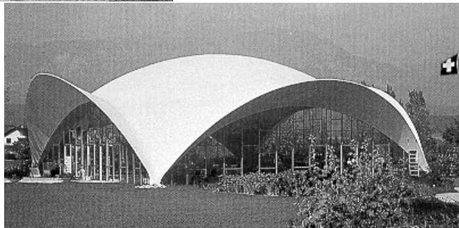
Centre de jardinage, Soleure, 1961 ing. H. Isler
